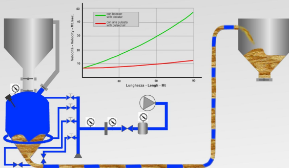
Schema tipico di impianto in fase pulsata Typical scheme of pulsed air plant
